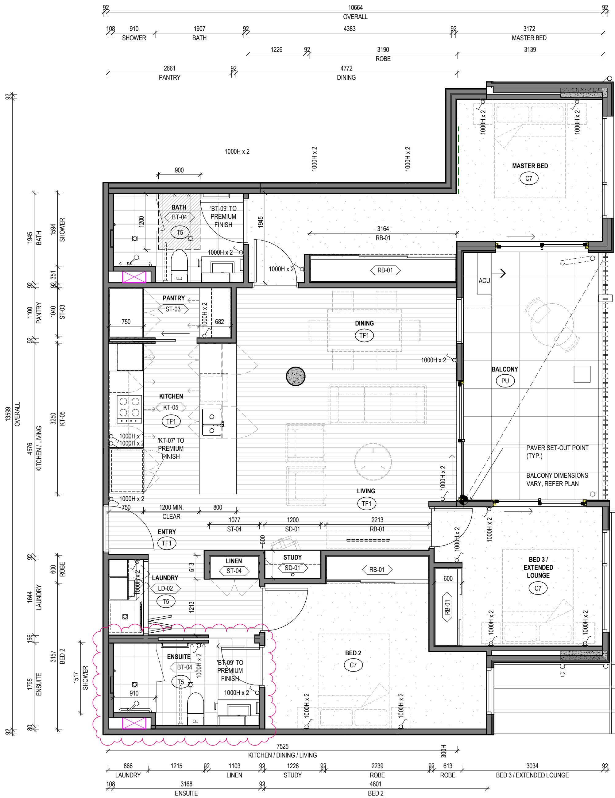
1 ILA Type 10 Scale 1 : 50
